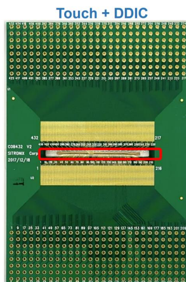
圖表一、矽創 TDDI
