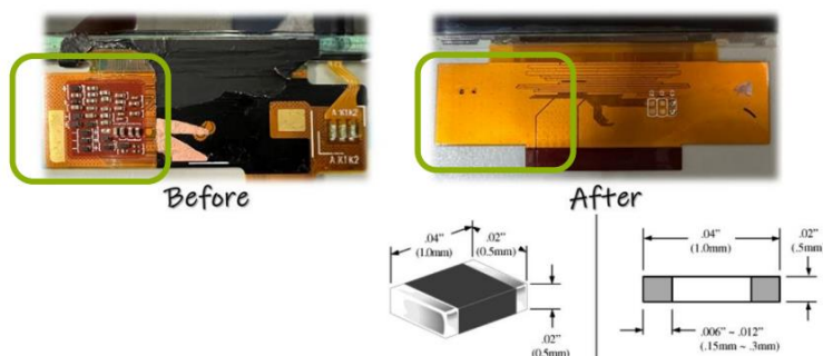
圖表二、減少外部電容，縮減厚度並達到窄邊框設計
